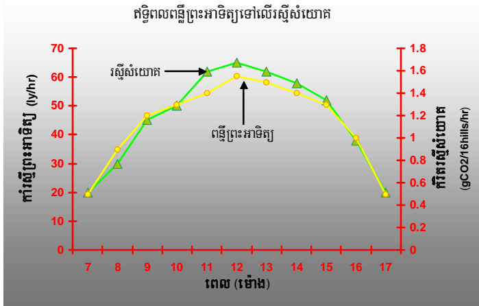
រូបភាព ២-១ ឥទ្ធិពលនៃពន្លឺព្រះអាទិត្យទៅលើការធ្វើរស្មីសំយោគ
