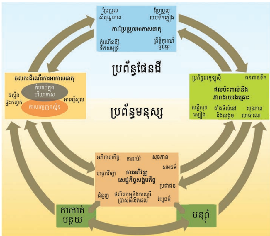
រូបភាព៤ សេចក្តីសង្ខេបបញ្ហាប្រែប្រួលអាកាសធាតុ
