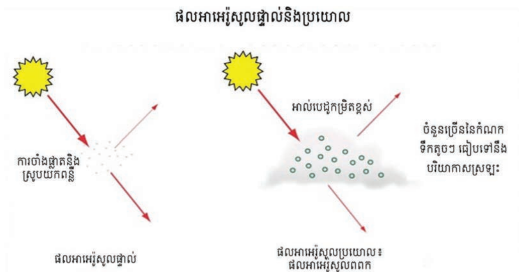
ដ្យាក្រាម១ ឥទ្ធិពលផ្ទាល់និងប្រយោលរបស់អាអេរ៉ូសូលទៅលើរំកាយរស្មីព្រះអាទិត្យ
