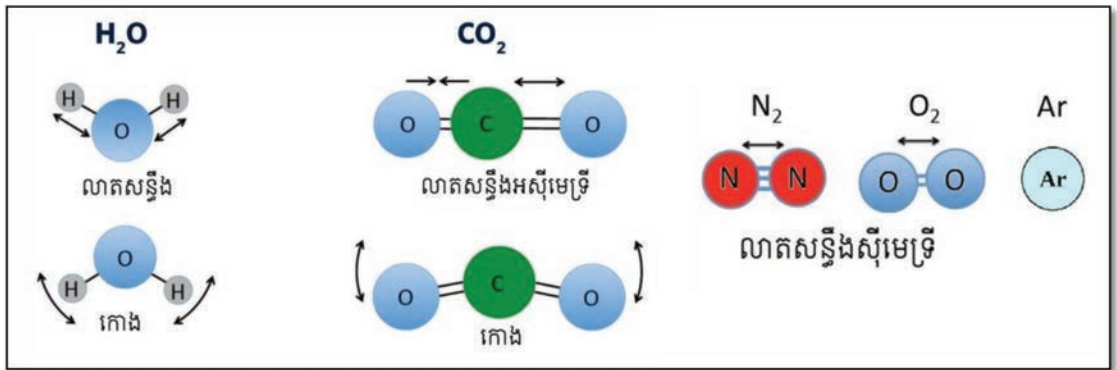
ដ្យាក្រាម២ ចលនាអាតូមរបស់ឧស្ម័នផ្ទះកញ្ចក់
