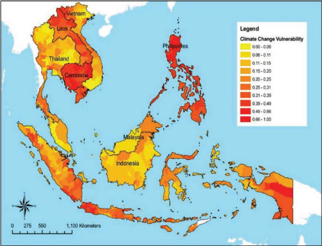
រូបភាព២ អនុគមន៍នៃភាពងាយរងគ្រោះនឹងការប្រែប្រួលអាកាសធាតុ
