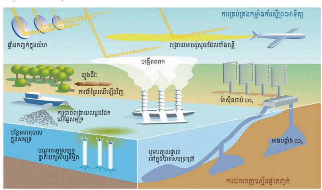
រូបភាព៨ វិស្វកម្មអាកាសធាតុ
