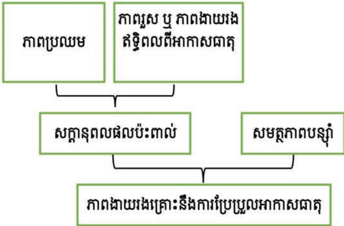
រូបភាព២ អនុគមន៍នៃភាពងាយរងគ្រោះនឹងការប្រែប្រួលអាកាសធាតុ
