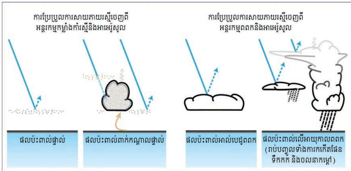
រូបភាព៤ តួនាទីរបស់អាអេរ៉ូសូលក្នុងបរិយាកាស
