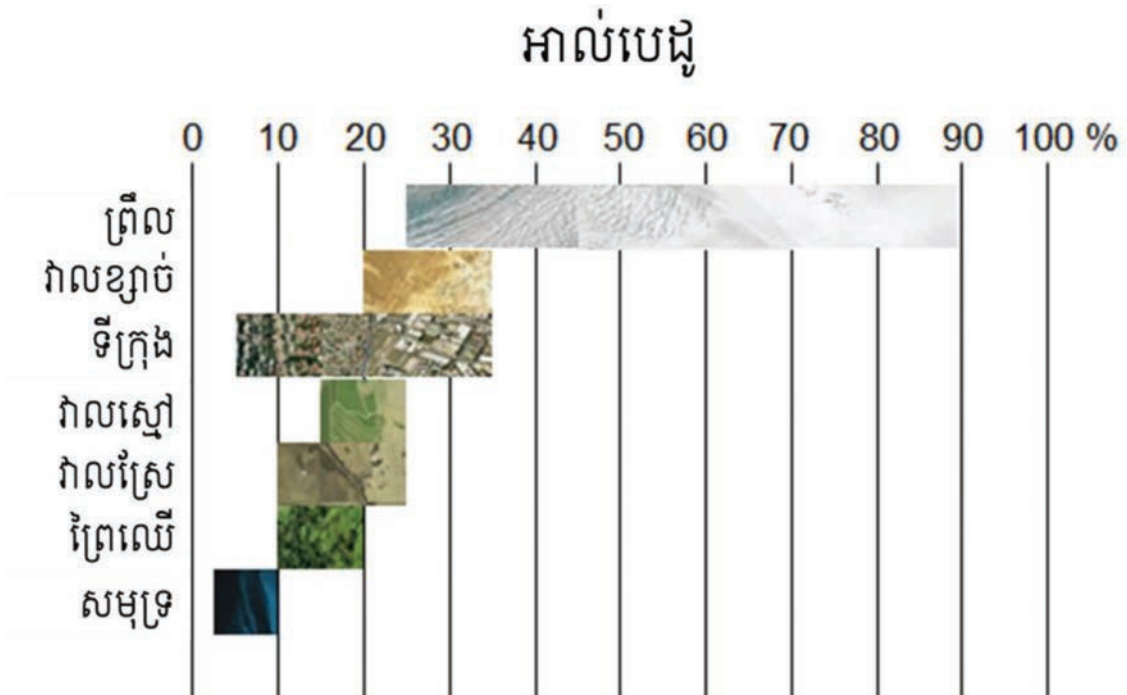
រូបភាព៥ កម្រិតអាល់បេដូផ្សេងៗ
