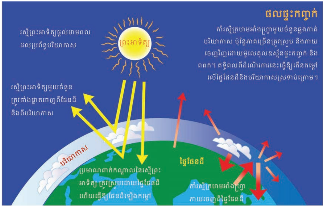
រូបភាព៦ បាតុភូតផលផ្ទះកញ្ចក់
