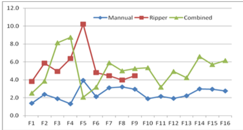
ក្រាហ្វិក៩. បរិមាណផលស្រូវគ្រុះបាត់នាពេលច្រូតកាត់ (y, %) ដោយការច្រូតដោយដៃ (Manual) ការច្រូតដោយម៉ាស៊ីន កាត់ផ្តុក (Ripper) និងច្រូតដោយម៉ាស៊ីនកុំប៉ែន (Combine harvester) ដែលវាស់វែងនៅស្រែចំនួន១៦ (F1-F16)
